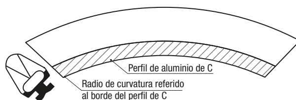
Figura "B" | Para bordes "B1NC" - "B1NC-AG" - "B2C" - "B2C-AG" - "B0C" - "B0C-AG"
