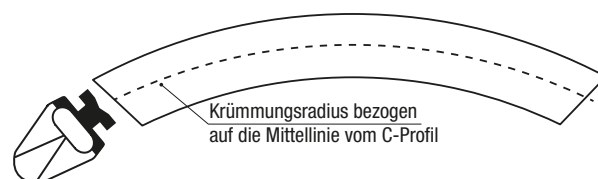
Bild "B" | Für Ränder "B1NC" - "B1NC-AG" - "B2C" - "B2C-AG" - "B0C" - "B0C-AG"
