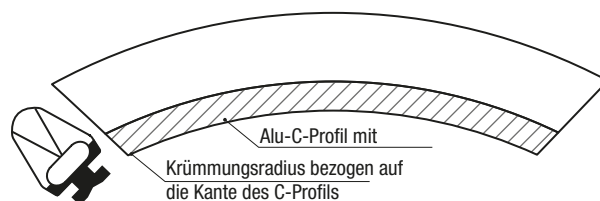
Bild "B" | Für Ränder "B1NC" - "B1NC-AG" - "B2C" - "B2C-AG" - "B0C" - "B0C-AG"
