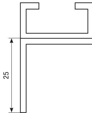
Tipo "SAL" | Perfil de "L" | para bordes tipo B2N
