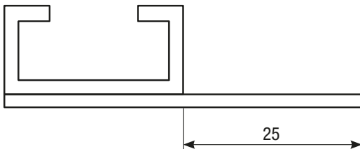
Tipo "SAI" | Perfil de "I" | para bordes tipo B2N
