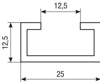
Tipo "SAC25" | Perfil de "C" | para bordes tipo B2N
