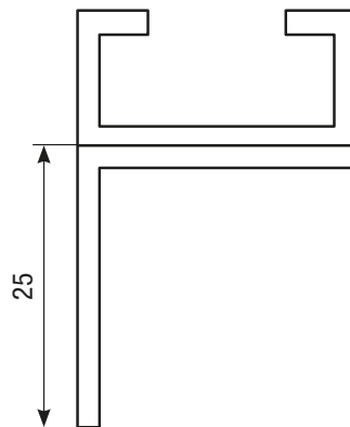
Tipo "SAL" | Profil en "L" | pour bords type B1N
