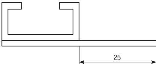
Tipo "SAI" | Profil en "I" | pour bords type B1N
