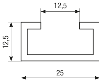
Tipo "SAC25" | Profil en "C" | pour bords type B1N
