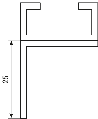
Tipo “SAL” | Perfil de “L” | para bordes tipo B1N
