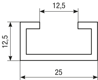
Tipo “SAC25” | Perfil de “C” | para bordes tipo B1N
